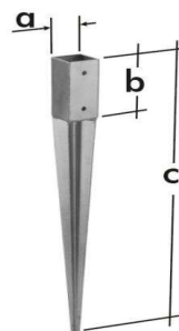
Kotviaci hrot - štvorcový žiarový zínok
