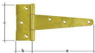
Záves trojuholníkový ZT zinok
