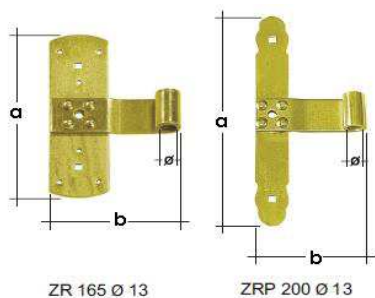
Záves križový ZR zinok
