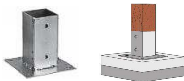
Kaslík na platničke štvorcový zínok
