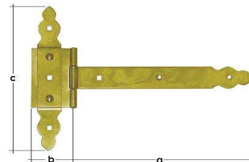
Záves bránkový ozdobný ZBNO zinok
