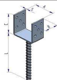
Kotvenie U úzke 200
