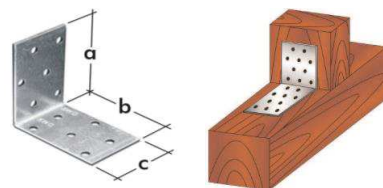
Uholník montážny KM zinok
