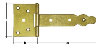
Záves bránkový ozdobný ZBO zinok
