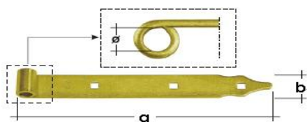
Záves pásový ZP zinok
