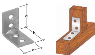
Uholník KW zinok
