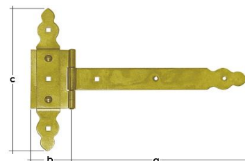
Záves bránkový ozdobný ZBNO zinok
