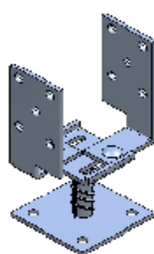
Kotvenie U šírkovo prestaviteľné s platňou šírka plechu 60mm, hrúbka 4mm roxor 18x100, zinok biely
