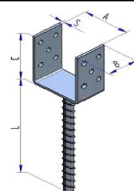
Kotvenie U úzke 200
