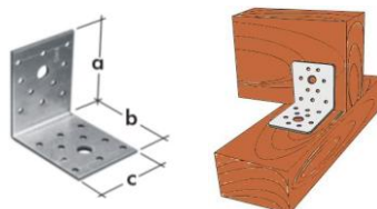
Uholník bez prelisu KL zinok
