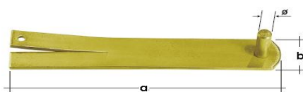
Držiak čapu do muriva CW zinok
