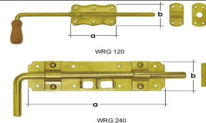
Zástrč zasúvací WRG zinok
