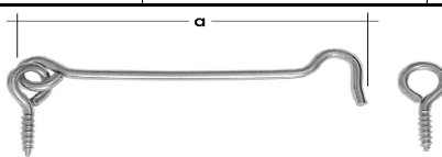
Háčik s očkom ZHK zinok
