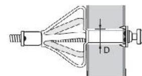
Hmoždinka oceľová-MOLLY do sadrokartónu a iných krehkých materiálov 4x25 P01300004025 4x38 P01300004038 4x45 P01300004045 4x52 P01300004052 4x65 P01300004065 5x45 P01300005045 5x58 P01300005058 5x71 P01300005071 5x88 P01300005088
