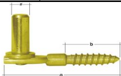
Držiak čapu CW zinok
