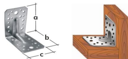
Uholník s prelisom KPW zinok
