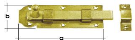
Zástrč jednoduchá W zinok
