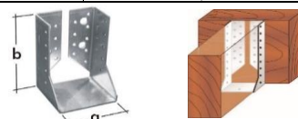
Papuče trámov vnútorné uzatvorenie zinok
