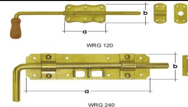
Zástrč zasúvacia WRG zinok
