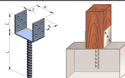
Kotvenie U úzke 200 A,B-vid tab.,C-105,S-4mm, L-200 mm zinok biely + lak
