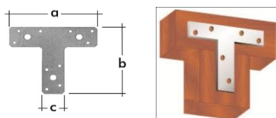
Spojovač T zinok
