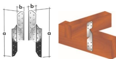
Krovová spojka zinok
