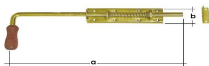
Zástrč pružinová s drev. koncovkou WSP zinok
