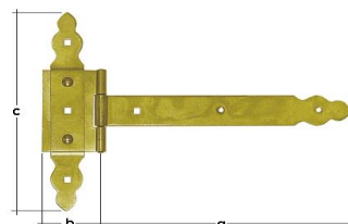
Záves bránkový ozdobný ZBNO zinok
